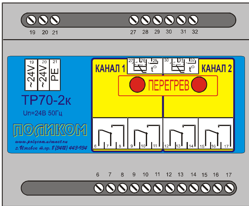
Рис. 1. Внешний вид термореле ТР70-2к.
